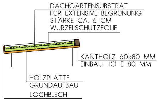
DACHBEGRUNUNG EINFACHE AUSFUHRUNG SCHNITT
